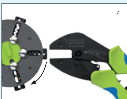
1–6: Быстрая смена плашек без вспомогательного инструмента – просто защелкнуть и готово! 1–6: Fast, tool-free die change - one click and you're done
