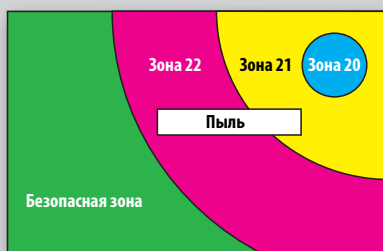
Пример типичного распределения зон при наполнении зернохранилища зерном.
